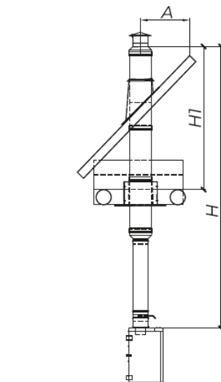
Дымоходная система внутри
