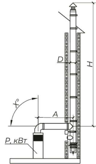
Дымоходная система внутри
