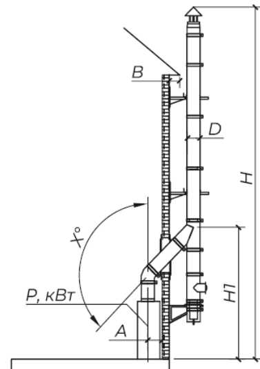
Дымоходная система снаружи
